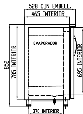
SECCIÓN SIN ENCIMERA
