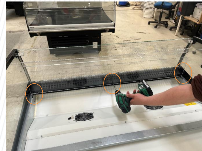
Billede 5: Indvendig plexiglas afmonteres
