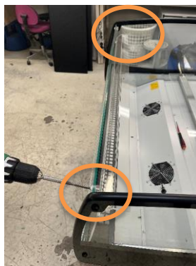
Billede 8: sideglasset afmonteres ved at fjerne skruerne
